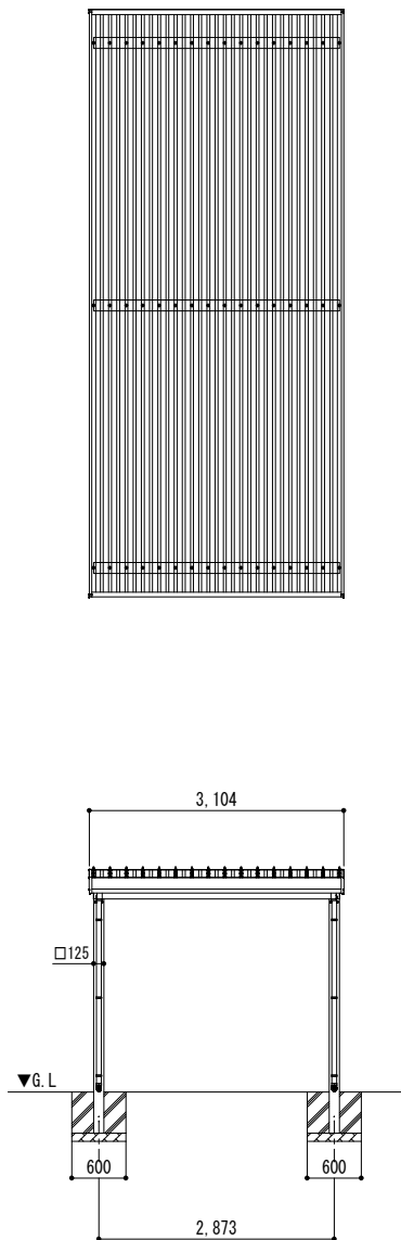
■ 姿図
