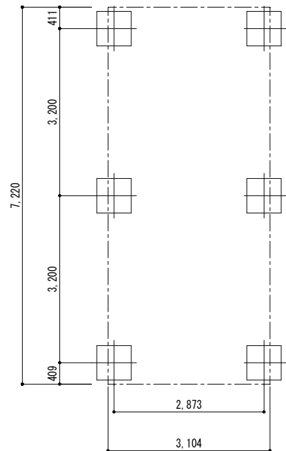
■ 基礎配置図
